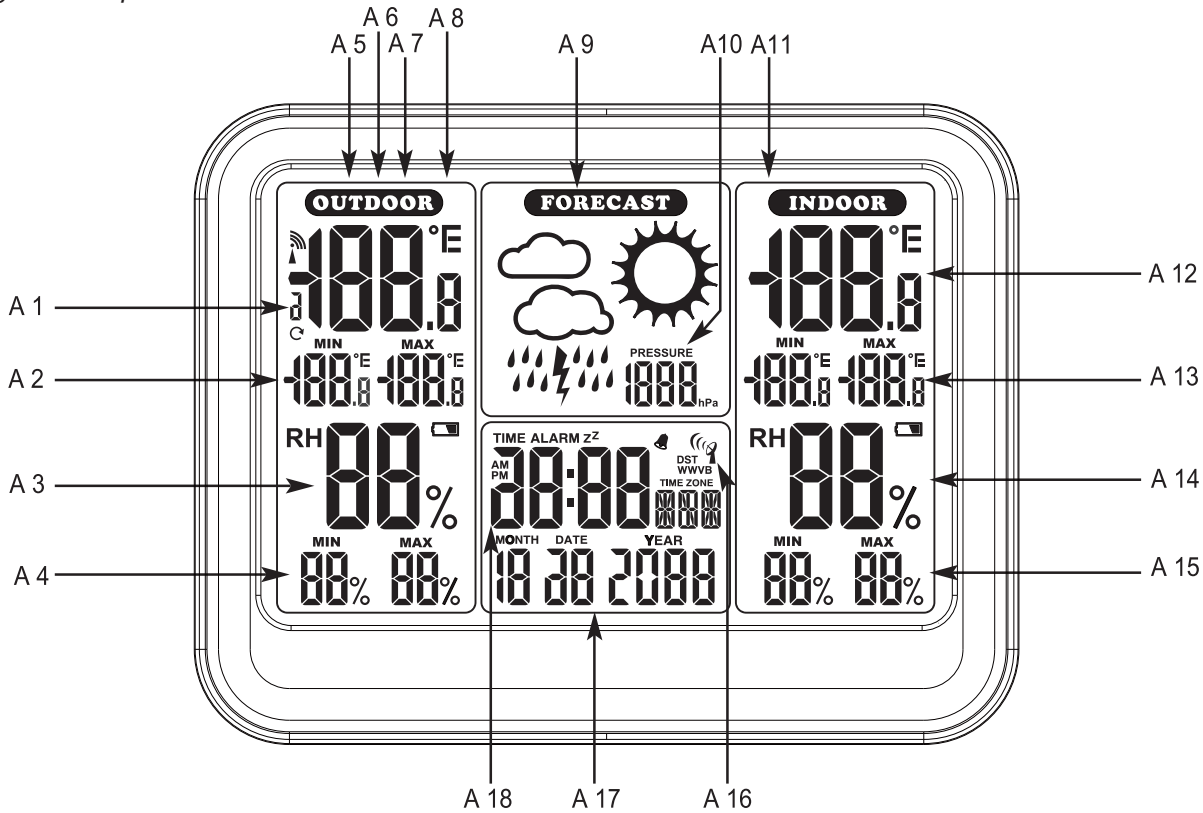
Fig. 1: Récepteur
