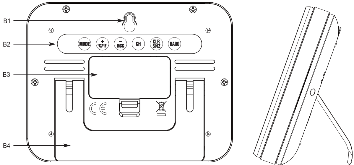
Fig. 2 : Récepteur
